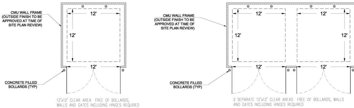
7 DUMPSTER LAYOUT DETAIL N.T.S.
